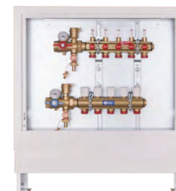
R553FKA Kompletní rozdělovač R553F s kulovými kohouty, vypouštěním, odvzdušněním a skříní do zdi.
